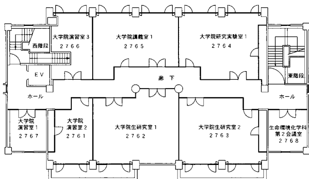
6階 平面図
