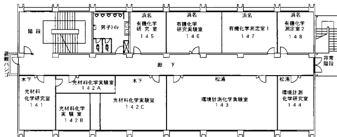
4階 平面図
