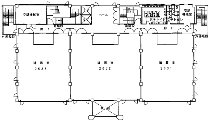
3階 平面図
