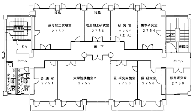
5階 平面図
