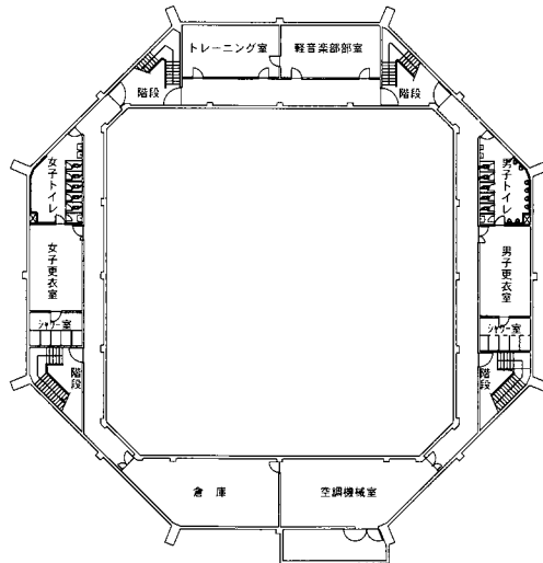
地階 平面図
