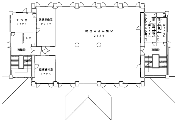
2階 平面図
