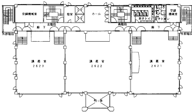
2階 平面図
