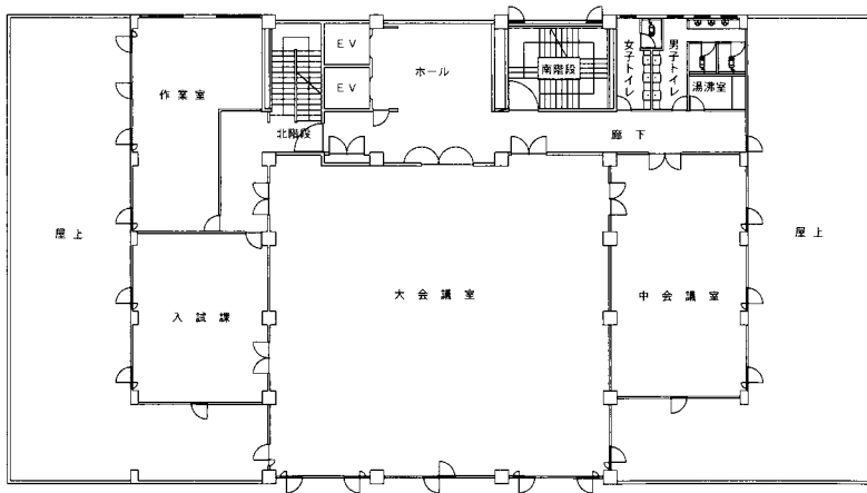
4階 平面図
