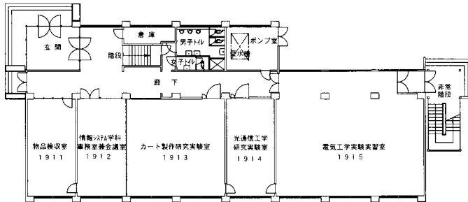
1階 平面図
