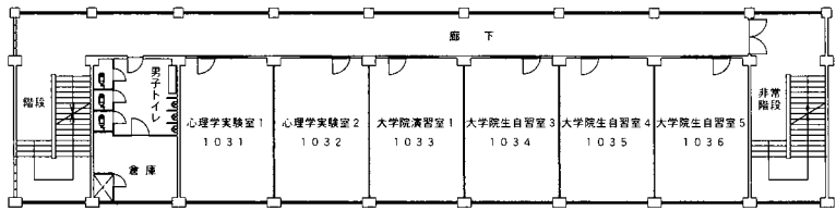
3階 平面図
