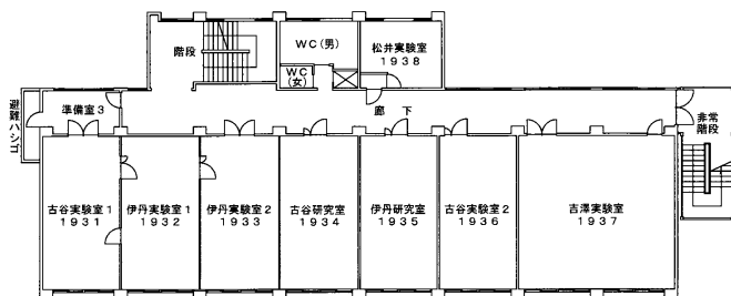
3階 平面図
