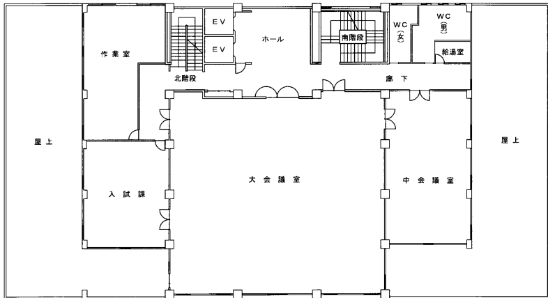
4階 平面図
