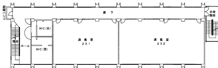
3階 平面図
