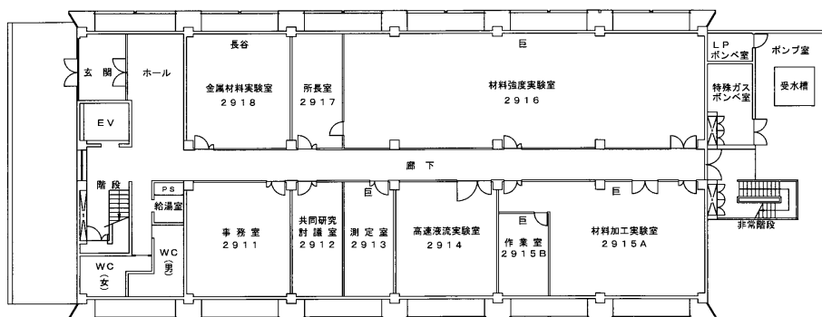
1階 平面図
