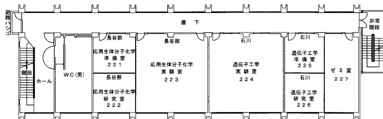
2階 平面図
