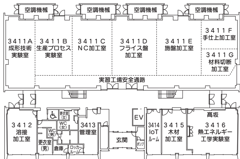
1階 平面図
