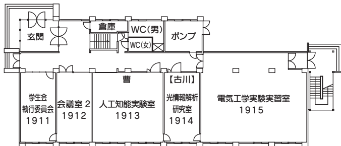
1階 平面図
