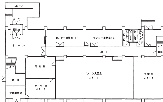
1階 平面図
