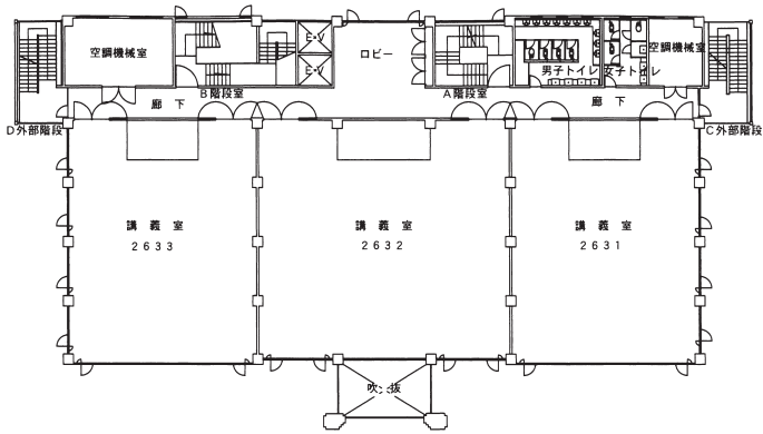
3階 平面図
