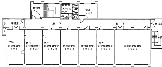
3階 平面図
