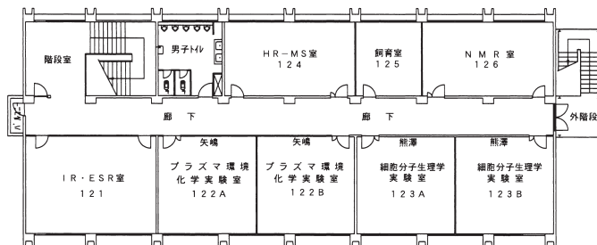
2階 平面図
