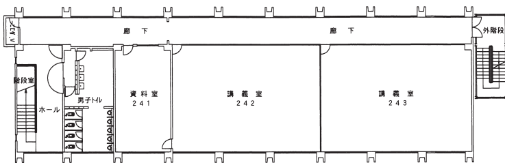
4階 平面図
