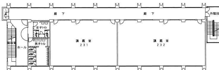
3階 平面図
