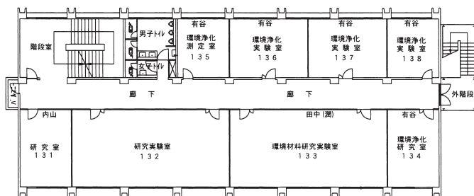
3階 平面図
