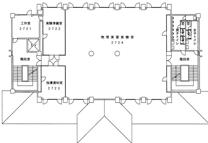
2階 平面図
