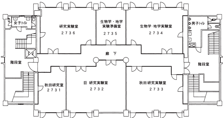
3階 平面図
