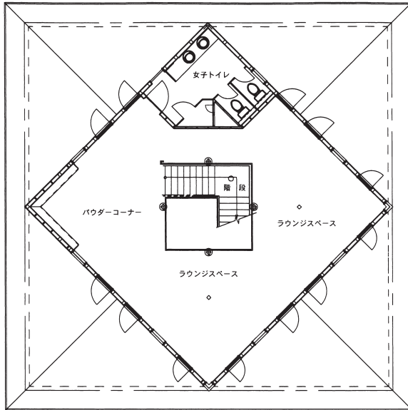
2階 平面図
