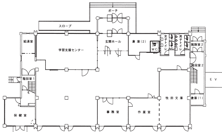
1階 平面図
