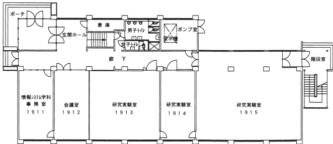
1階 平面図
