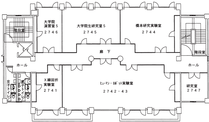
4階 平面図
