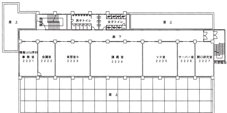
2階 平面図
