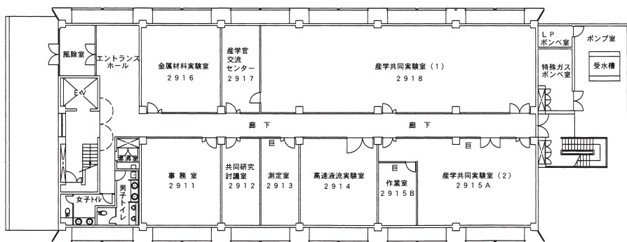
1階 平面図
