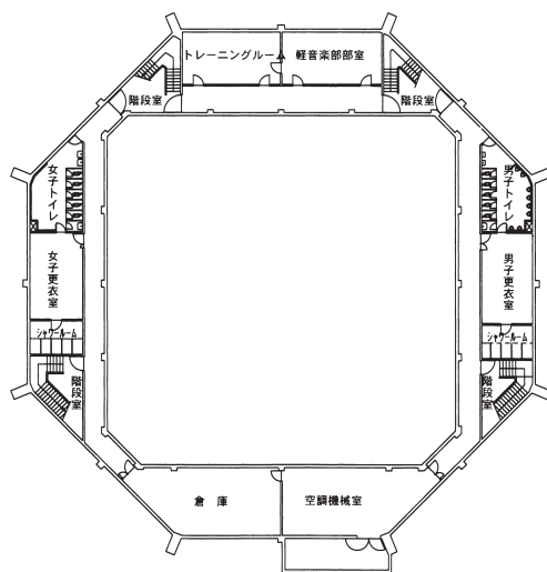
地階 平面図
