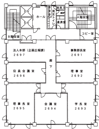
9階 平面図
