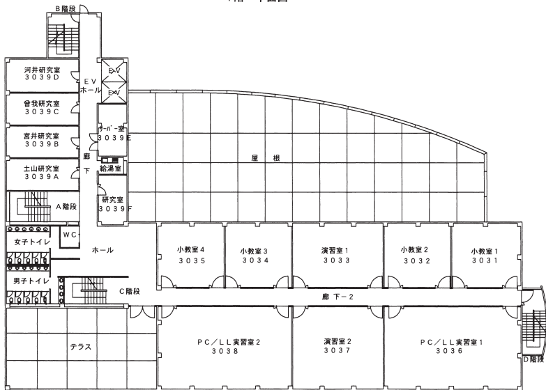
4階 平面図
