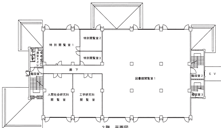
2階 平面図
